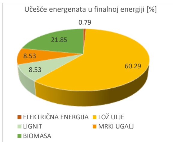
Dijagram 5-20: Udio razmatranih energenata u potrebnoj finalnoj energiji za grijanje javnih zgrada koje nijesu u vlasništvu JLS u kontrolnoj godini
