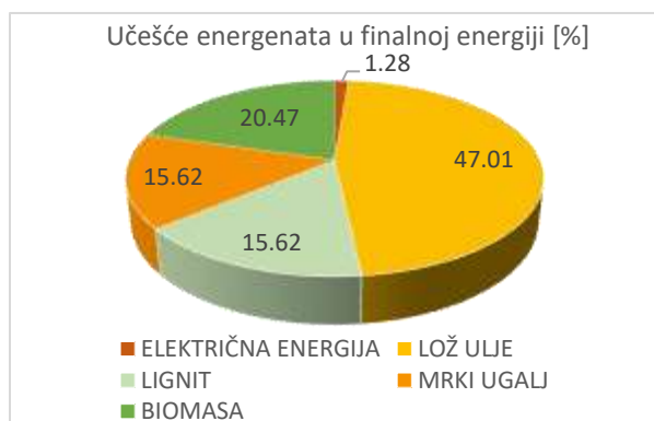
Dijagram 5-3: Udio razmatranih energenata u potrebnoj finalnoj energiji za grijanje javnih zgrada koje nijesu u vlasništvu JLS u baznoj godini
