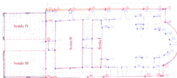
Основа цркве са положајем испитних сонди
