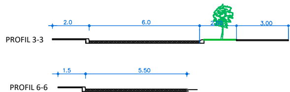
KARAKTERISTIČNI POPREČNI PROFILI 1:100
